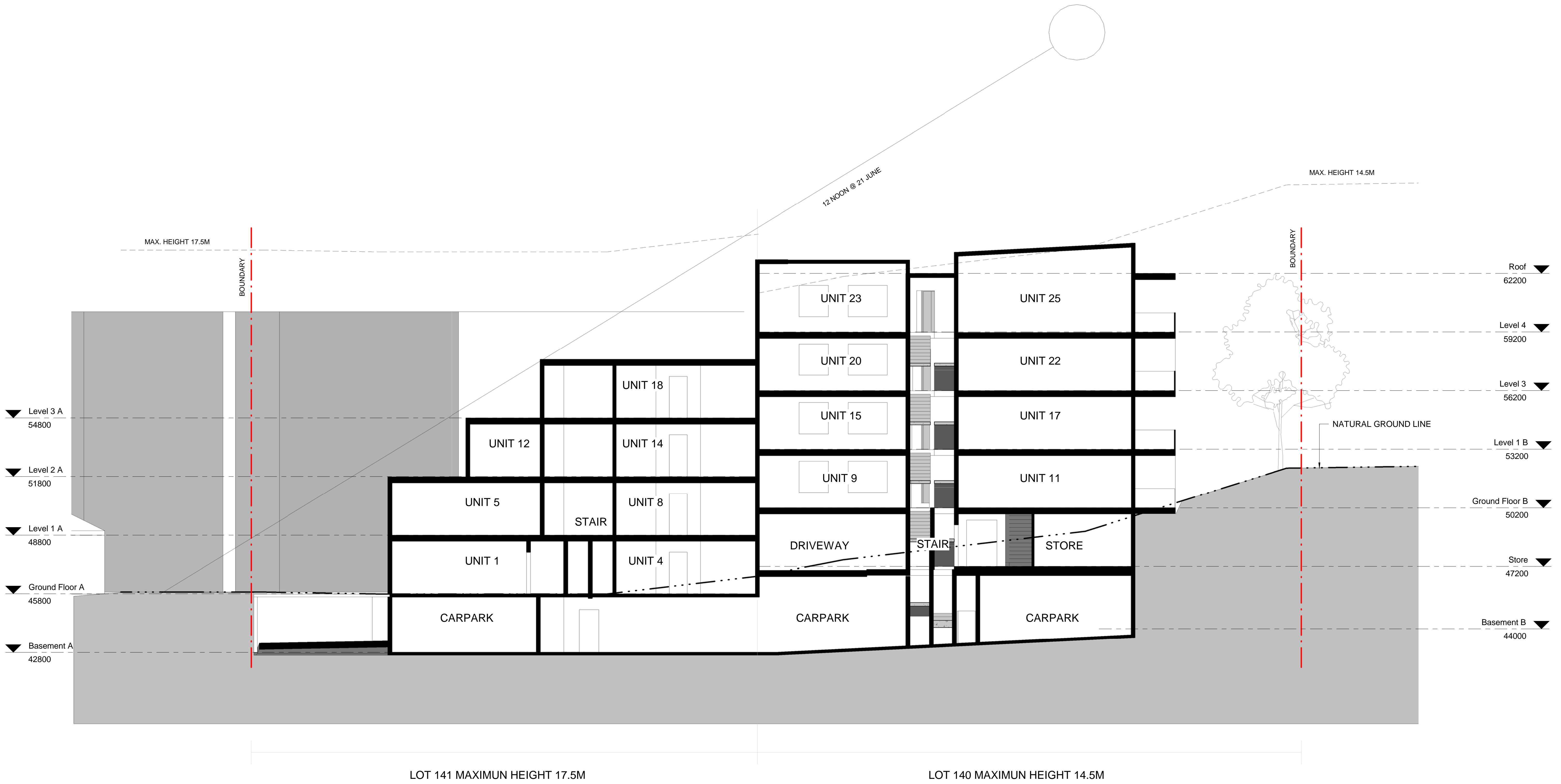
1 Section 1 1 : 100
